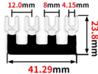
38637-TS 4 Pos
