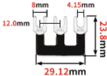
38636-TS 3 Pos
