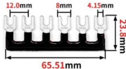
38639-TS 6 Pos
