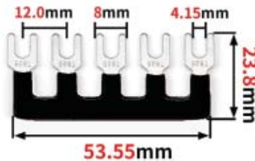
38638-TS 5 Pos
